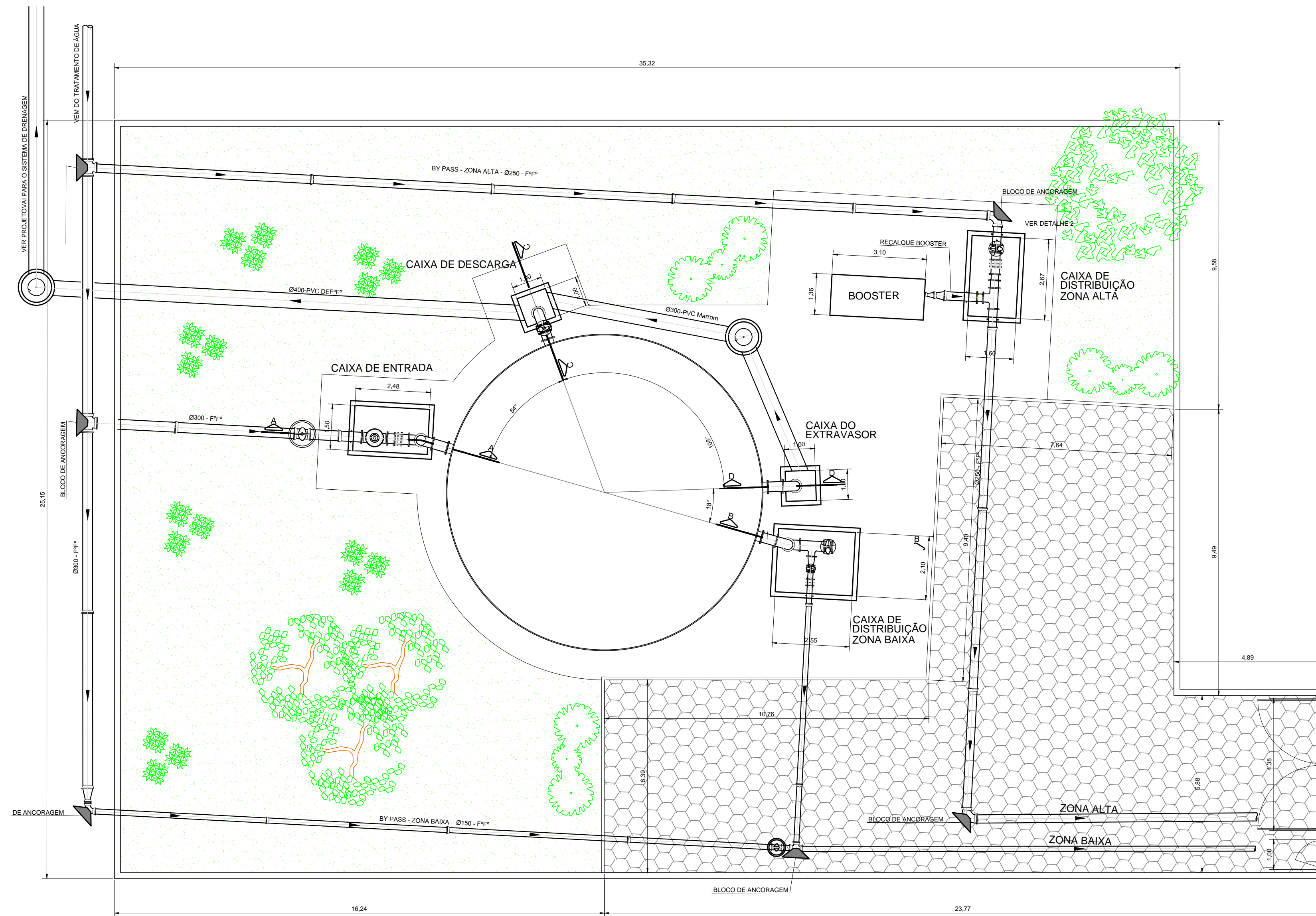
PLANTA ESC. 1:100
