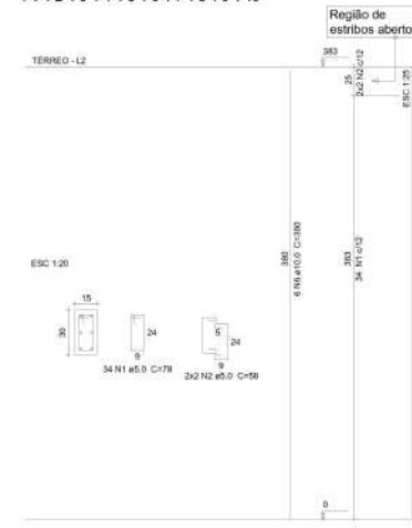
PILAR escala: indicada
