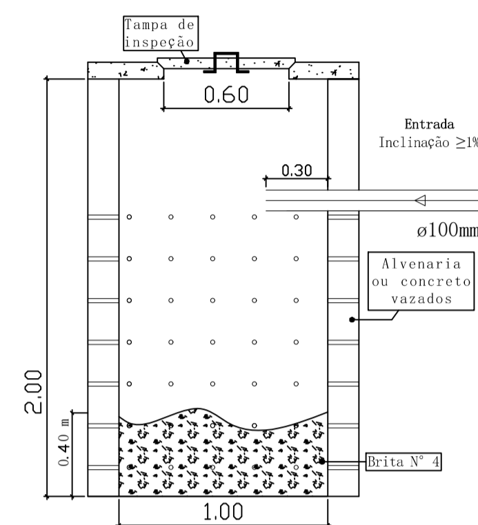
Sumidouro CORTE 1-1
