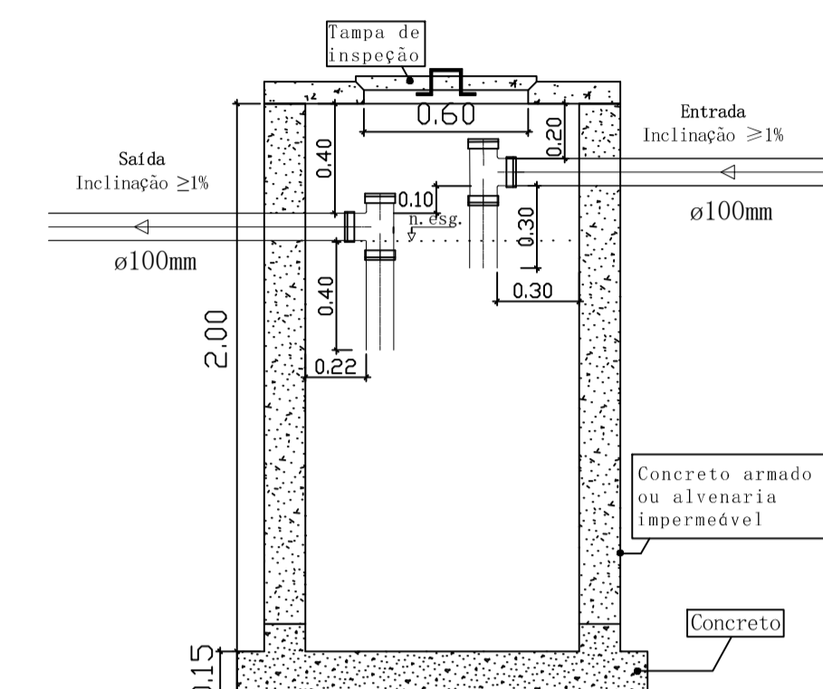
Fossa séptica CORTE 2-2
