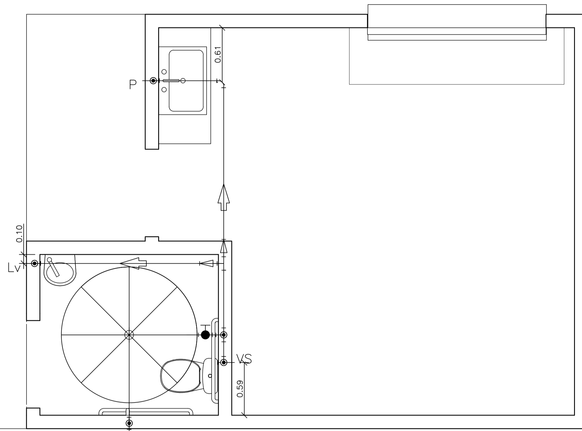
DETALHE DAS INSTALAÇÕES DOS APARELHOS SANITÁRIOS ACESSÍVEIS
