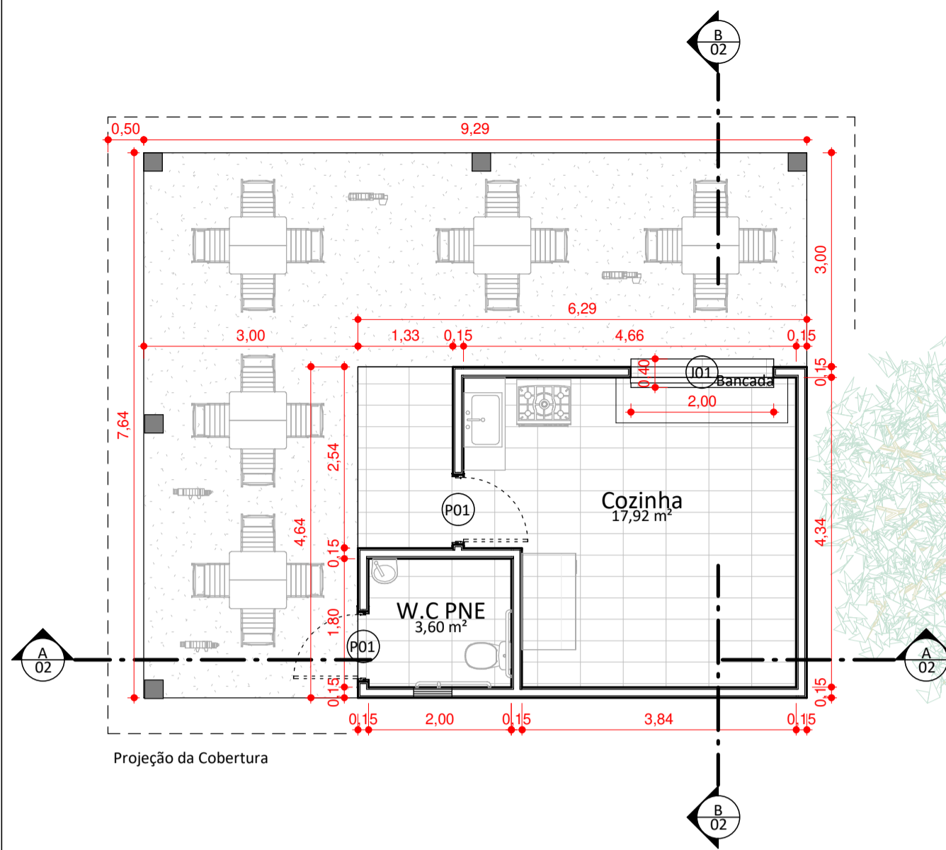
1 Planta Baixa 1:75
